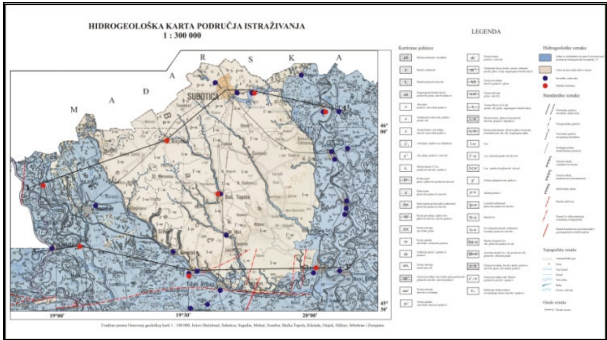
Slika 2: Hidrogeološka karta područja istraživanja
